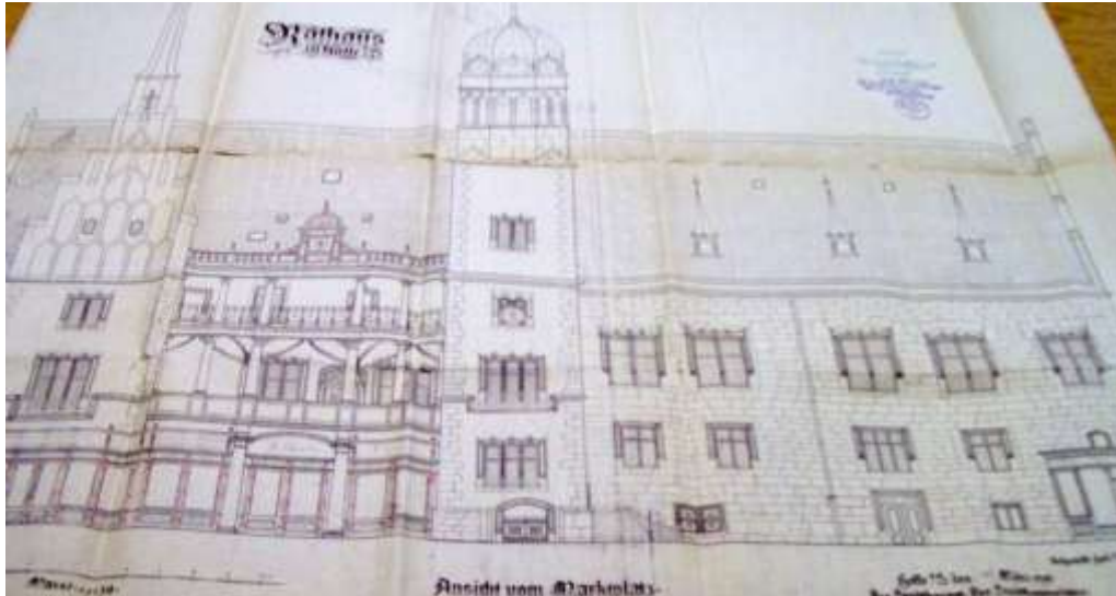
Amtliche Fassadenzeichnung des Alten Rathauses, 1919 – Quelle: Stadtarchiv Halle (Saale)
